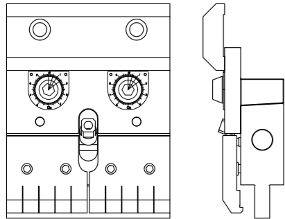
安全快速夾具系統 (手動) Quick-release Safety Clamp (Manual)
