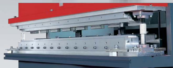
平面抽折專用模具 Deflection Control Die
